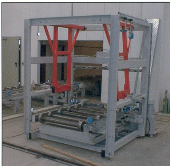
Stapelmagazin für Europaletten
